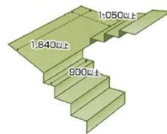
踊り場の許容寸法(mm)
